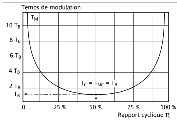
Temps de modulation du «Train d'ondes» en fonction de la consigne
