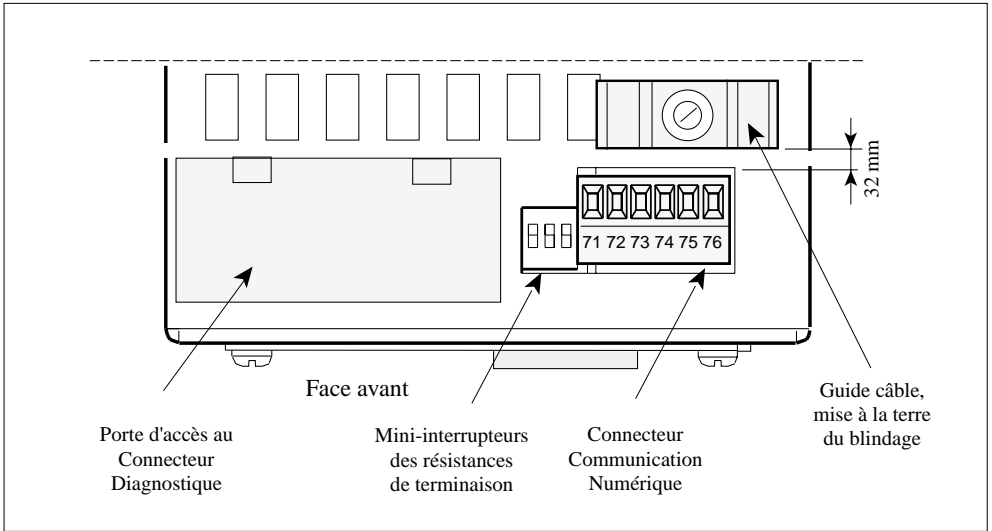
Figure 3-5 Disposition en option du bornier Communication Numérique (calibres 16 à 100A) Vue de dessus
