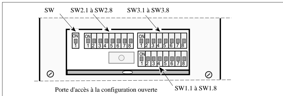
Figure 6-2 Mini-interrupteurs de configuration de fonctionnement (vue de la face avant)
